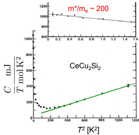
Abbildung 5.17: Wärmekapazität als Funktion der Temperatur für Metalle mit 4f und 5f Elektronen.
