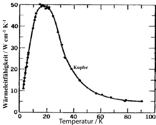
Abbildung 5.31: Temperaturabhängigkeit der Wärmeleitfähigkeit von Kupfer.
