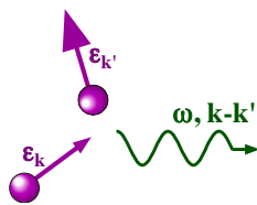
Abbildung 5.22: Elektron-Phonon Streuung.
