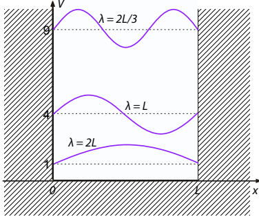
Abbildung 5.6: Eindimensionaler Potentialtopf.
