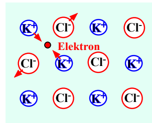
Abbildung 5.46: Gitterverzerrung durch Wechselwirkung mit Elektron.
