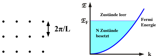
Abbildung 5.7: Links: Zustände im k -Raum; rechts: Besetzung der Zustände bei T = 0 .
