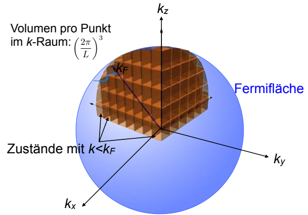
Abbildung 5.8: Fermikugel.
