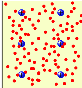
Abbildung 5.41: Elektronengas.
