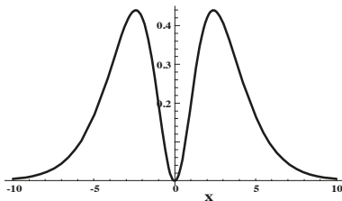
Abbildung 5.14: Grafische Darstellung des Integranden in Gl. (5.10).
