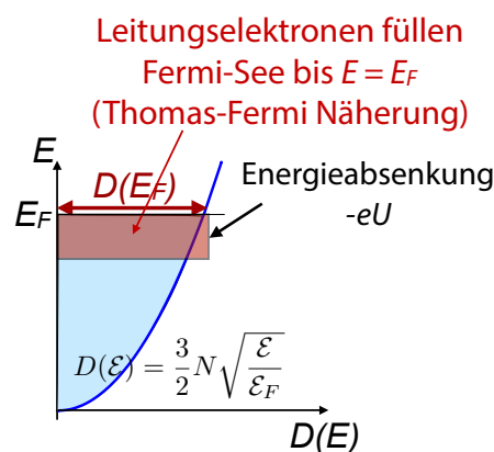
Abbildung 5.37: Abschätzung der zusätzlichen Ladungsdichte.
