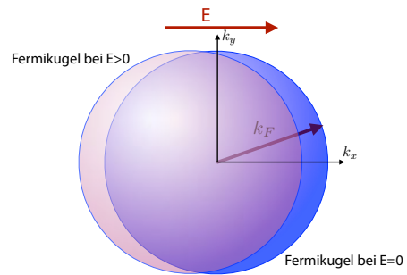
Abbildung 5.19: Verschobene Fermikugel im elektrischen Feld.
