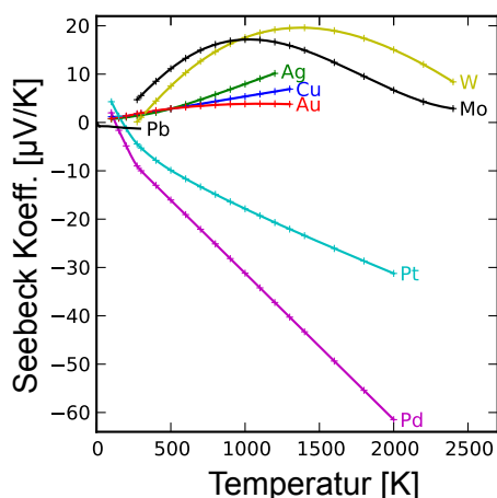
Abbildung 5.35: Seebeck-Koeffizienten unterschiedlicher Metalle als Funktion der Temperatur.
