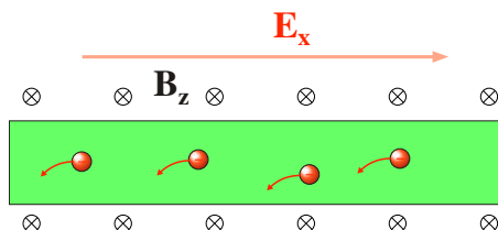
Abbildung 5.26: Bewegung von Elektronen in gekreuzten E/B Feldern.
