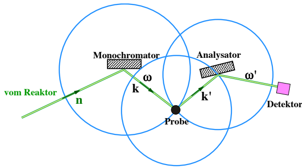
Abbildung 4.42: 3-Achsen Neutronenspektrometer.
