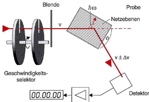
Abbildung 4.43: Flugzeit-Spektrometer für Neutronen.
