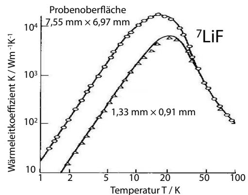
Abbildung 4.81: Temperaturabhängigkeit des Wärmeleitkoeffizienten in unterschiedlichen Proben.
