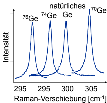
Abbildung 4.40: Raman-Streuung an Germanium mit unterschiedlichen Atommassen.
