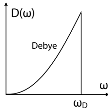
Abbildung 4.53: Zustandsdichte im Debye-Modell.
