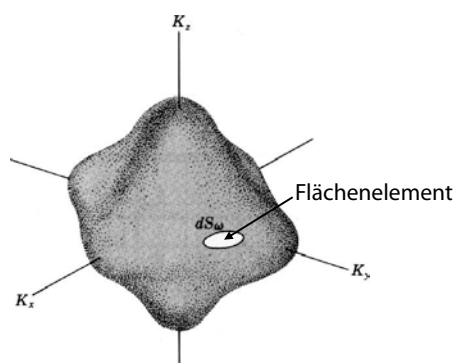
Abbildung 4.63: Isfrequenzfläche in 3D.
