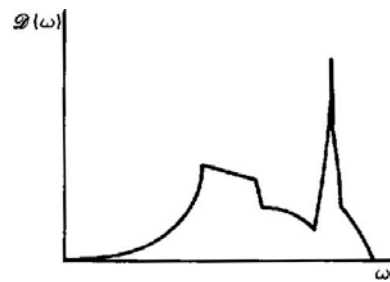
Abbildung 4.60: Reale Zustandsdichte.
