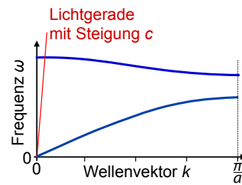
Abbildung 4.36: Vergleich der Dispersion von Phononen und Schwingungsmoden.
