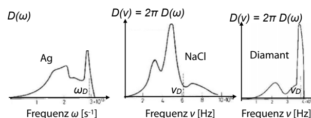
Abbildung 4.65: Zustandsdichten für Silber, Kochsalz und Diamant.
