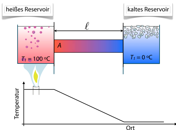
Abbildung 4.73: Wärme wird über einen Stab zwischen 2 Wärmereservoirs übertragen.
