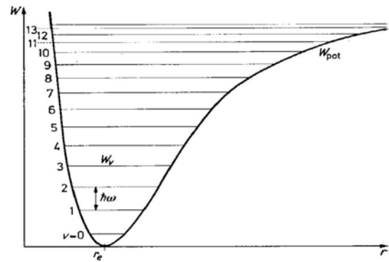
Abbildung 4.67: Anharmonisches Potenzial.
