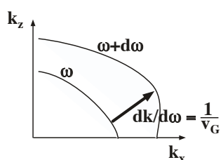
Abbildung 4.62: Abstand zwischen Iso-Frequenzflächen.
