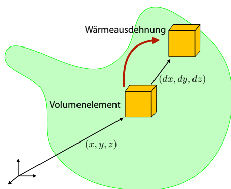
Abbildung 4.69: Wärmeausdehnung.
