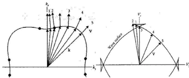
Abbildung 4.19: Links: Oberfläche konstanter Frequenz im k -Raum und zugehörige Gruppengeschwindigkeitsvektoren. Rechts: Wellenfront und Ausbreitungsrichtung.
