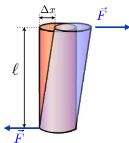
Abbildung 4.14: Scherung.
