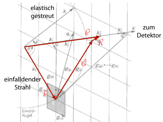
Abbildung 4.41: Impulse beim inelastischen Streuprozess.
