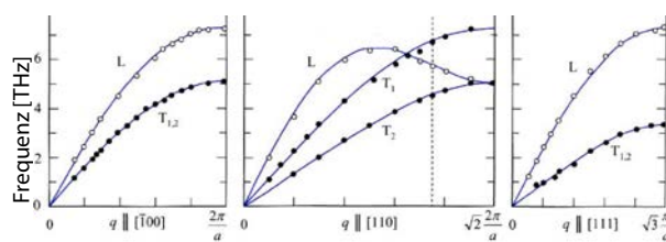
Abbildung 4.32: Phononenspektrum für Kupfer.
