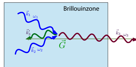
Abbildung 4.76: Umklapp-Prozess.
