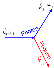
Abbildung 4.37: Inelastische Lichtstreuung.
