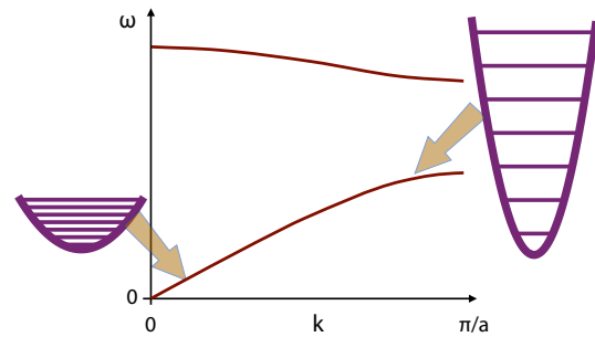
Abbildung 4.47: Zwei unabhängige Phononenfreiheitsgrade.
