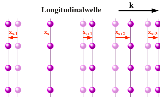
Abbildung 4.23: Longitudinalwelle.
