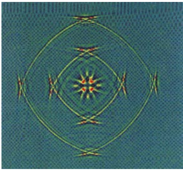
Abbildung 4.18: Experimentell gemessene Wellenfronten in Si. Die drei Wellenfronten entsprechen unterschiedlichen Zeiten von 1,76, 2,04 und 2,42 \mu\text{s} . [20]
