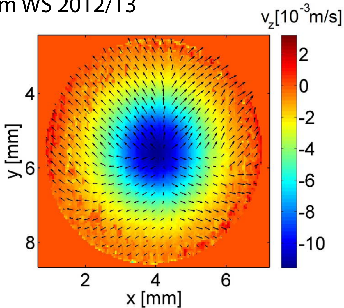
Gemessenes Strömungsprofil
