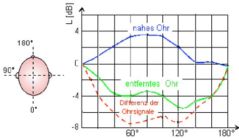
Abbildung 4.33: Interaurale Intensitätsdifferenz. [1]
