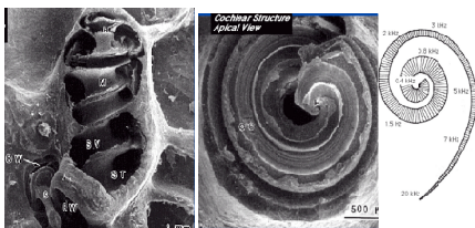
Abbildung 4.13: Cochlea (Schnecke).
