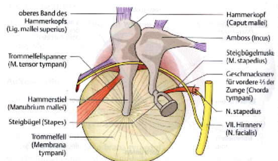
Abbildung 4.10: Mittelohr
