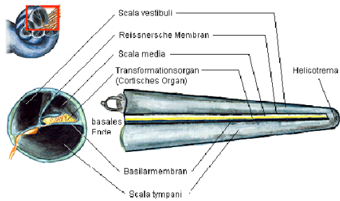
Abbildung 4.12: Innenohr. [1]
