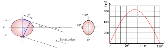
Abbildung 4.34: Laufzeitunterschiede. [1]
