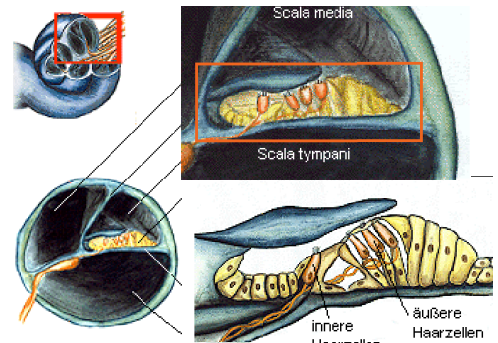
Abbildung 4.14: Transformationsorgan. [1]
