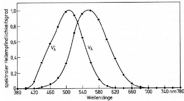
Abbildung 5.27: Relative spektrale Helligkeit des Auges für Tagessehen V(\lambda) und Nachtsehen V'(\lambda) . [4]
