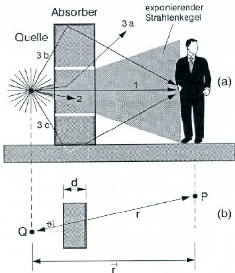
Abbildung 11.30: Abschirmung und Aufbaustrahlung.
