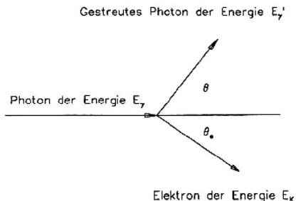
Abbildung 11.3: Compton Effekt.
