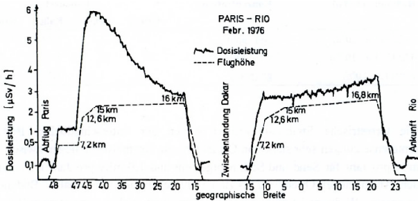
Abbildung 11.37: Höhenstrahlung.
