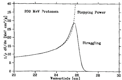
Abbildung 11.16: Tiefendosiskurve für 200 MeV Protonen in Wasser.
