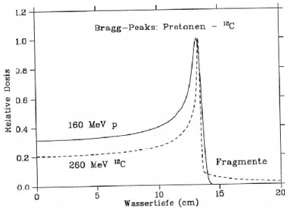
Abbildung 11.17: Tiefendosiskurve Protonen und 12 C.
