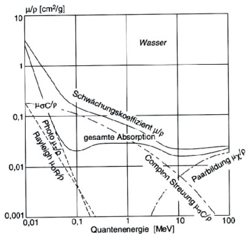
Abbildung 11.9: Massenschwächungskoeffizient von Wasser.
