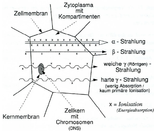
Abbildung 11.20: Ionisationsdichte.
