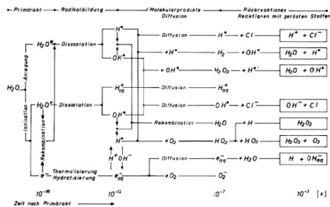
Abbildung 11.25: Indirekte Strahlenwirkung.
