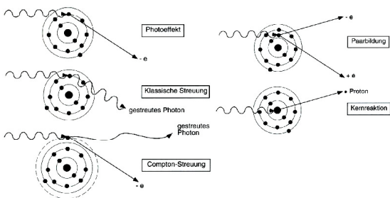
Abbildung 11.2: Primärprozesse Photonen.
