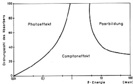
Abbildung 11.12: Dominanz verschiedener Effekte.
