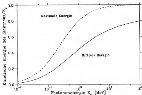
Abbildung 11.6: Kinetische Energie des Elektrons.
