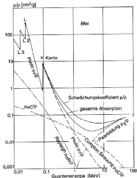
Abbildung 11.8: Massenschwächungskoeffizient von Blei.
