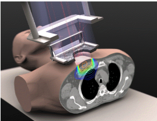
Abbildung 11.1: Strahlentherapie
