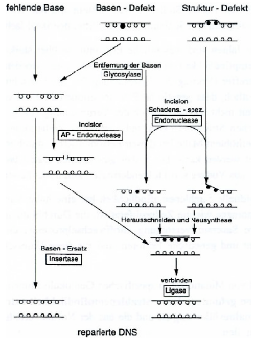
Abbildung 11.24: Enzymatische DNS-Reparatur.
