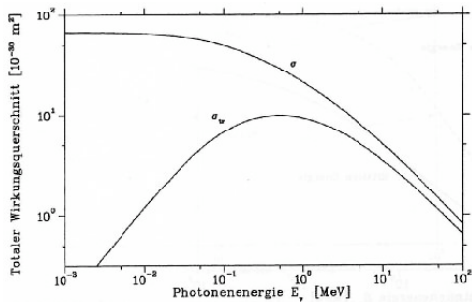
Abbildung 11.5: Energieaufteilung.
