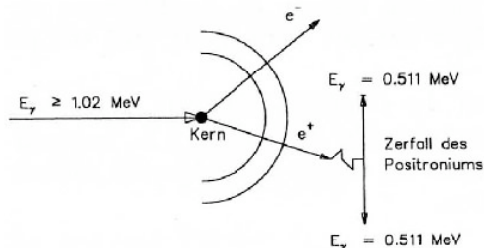
Abbildung 11.7: Paarbildung.
