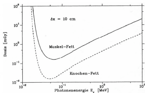
Abbildung 11.11: Dosisbelastung abhängig von der Photonenenergie.
