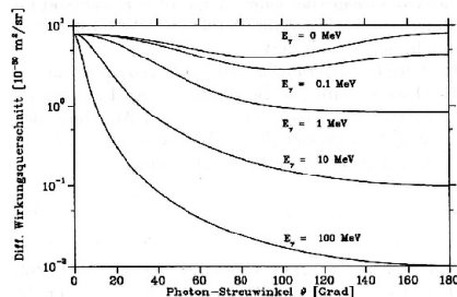
Abbildung 11.4: Streuwinkel.
