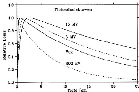
Abbildung 11.13: Tiefendosiskurven.
