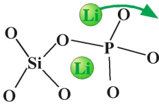
Abbildung 1.34: Hüpffprozesse von Li in \text{Li}_2\text{O-SiO}_2\text{-P}_2\text{O}_5 .
