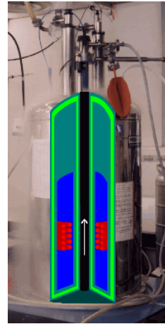
Abbildung 1.38: Supraleitender Magnet
