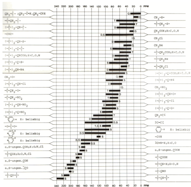
Abbildung 1.17: Übersicht über die wichtigsten Bereiche der chemischen Verschiebung von ^{13}C .
