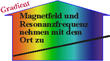
Abbildung 1.19: Ortsabhängige Resonanzfrequenz in einem inhomogenen Magnetfeld.
