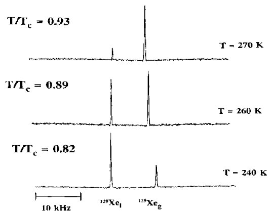
Abbildung 1.30: ^{129}\text{Xe} NMR von Gas und Flüssigkeit.
