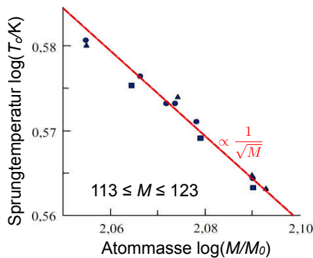
Abbildung 9.23: Kritische Temperatur von Zinn als Funktion der Atommasse.
