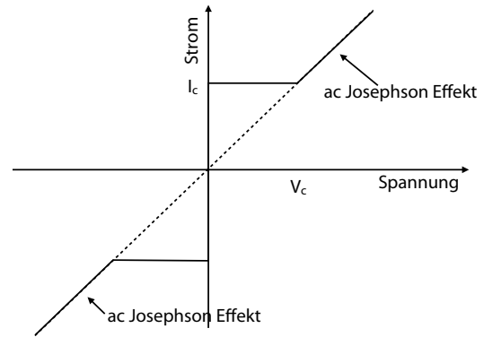
Abbildung 9.43: Strom-Spannung Kurve bei einem Josephson Kontakt.
