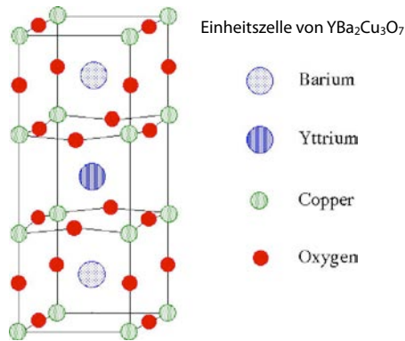
Abbildung 9.16: Typische Struktur eines Hochtemperatur-Supraleiters.
