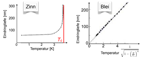
Abbildung 9.28: Eindringtiefe für Zinn und Blei als Funktion der Temperatur.
