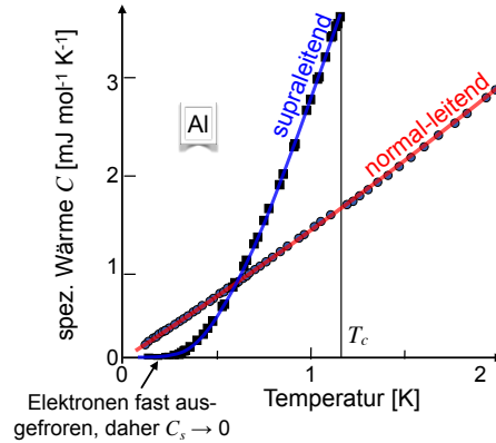
Abbildung 9.19: Temperaturabhängige spezifische Wärme von Aluminium.
