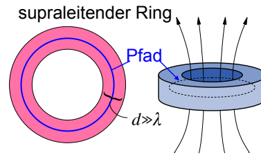
Abbildung 9.31: Geschlossener Pfad in einem supraleitenden Ring.
