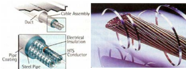
Abbildung 9.36: Supraleitende Drähte.
