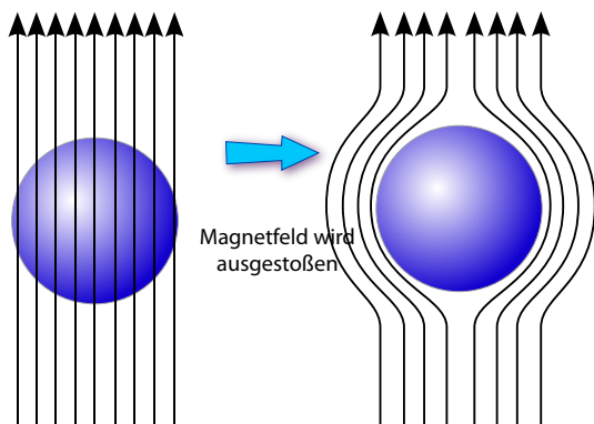
Abbildung 9.6: Meissner-Effekt: Ein Supraleiter ist ein perfekter Diamagnet.
