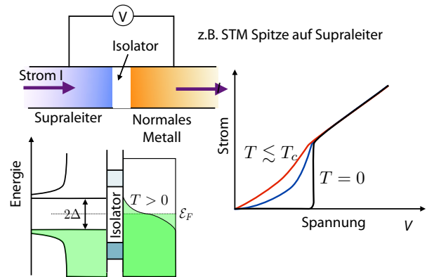
Abbildung 9.39: Tunnelkontakt zwischen Supraleiter und Normalleiter.
