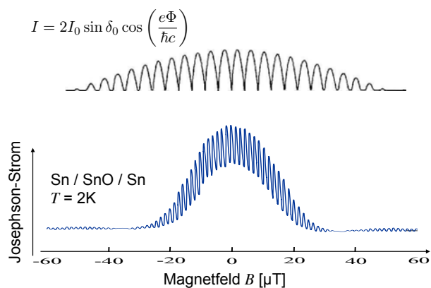
Abbildung 9.47: Oszillationen des maximalen Stroms durch ein SQUID als Funktion der Flussdichte.
