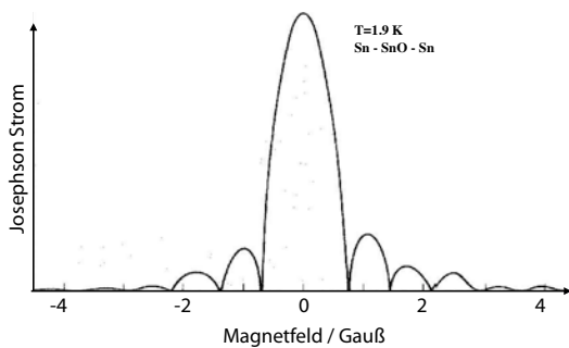
Abbildung 9.45: Abhängigkeit des Josephson Stroms von der Flussdichte.
