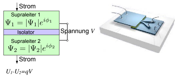
Abbildung 9.42: Josephson-Kontakt.
