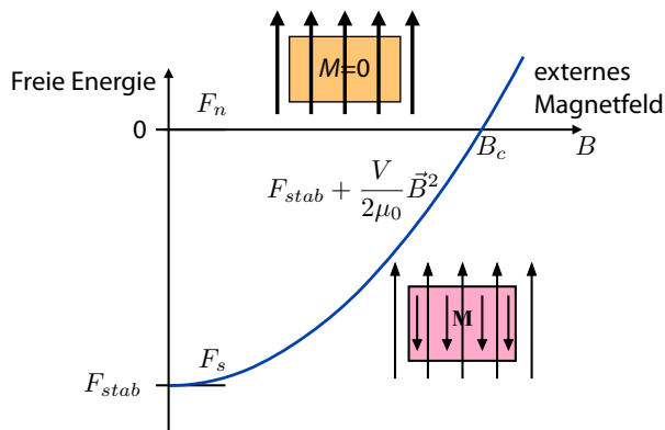
Abbildung 9.25: Energie des normalleitenden Zustandes ( F_n ) und des supraleitenden Zustandes ( F_s ) als Funktion der Stärke des externen Magnetfeldes.
