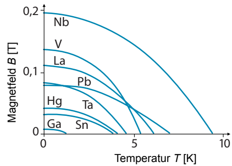
Abbildung 9.9: Temperaturabhängigkeit des kritischen Feldes bei Typ I Supraleiter.
