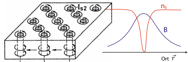
Abbildung 9.29: Flussschläuche mit Ringströmen (links) und Verlauf des Ordnungsparameters n_s in der Nähe eines Fluss Schlauches in einem Typ II Supraleiter (rechts).
