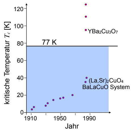
Abbildung 9.24: Maximale kritische Temperatur als Funktion der Zeit.
