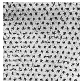
Abbildung 9.15: Hexagonales Gitter aus Flusssquanten.
