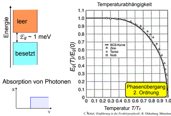
Abbildung 9.22: Energielücke, Temperaturabhängigkeit und Absorptionsspektrum.
