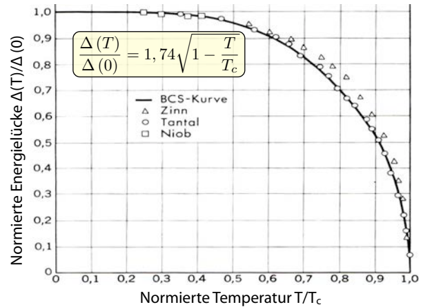
Abbildung 9.35: Normierte Energielücke als Funktion der Temperatur.
