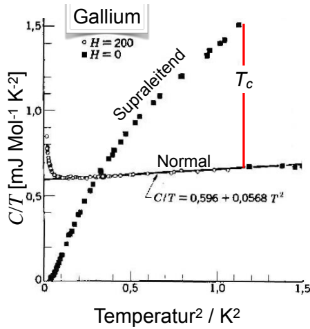
Abbildung 9.20: Temperaturabhängige spezifische Wärme von Gallium. [14]
