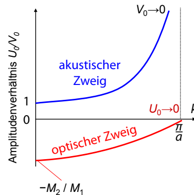
Abbildung 4.28: Schwingungsamplituden für den akustischen und den optischen Zweig als Funktion der Wellenzahl.
