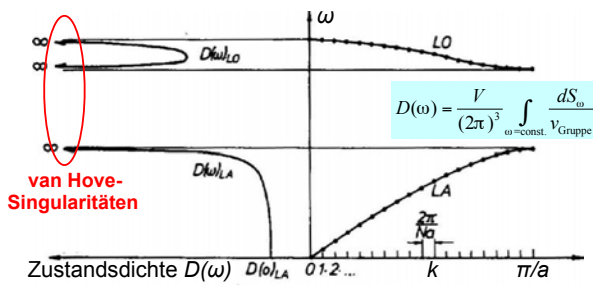
Abbildung 4.61: Zustandsdichte mit Singularitäten für ein einfaches Modell.
