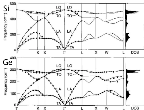
Abbildung 4.64: Dispersion und Zustandsdichte für Si und Ge.
