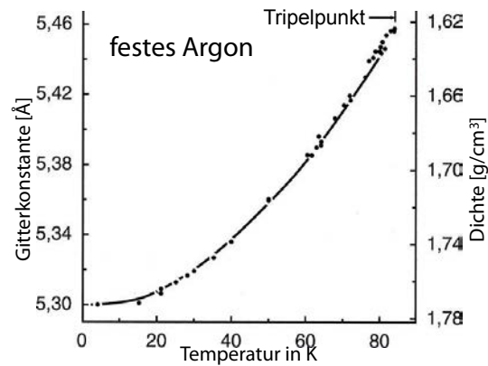
Abbildung 4.68: Wärmeausdehnung von festem Argon.
