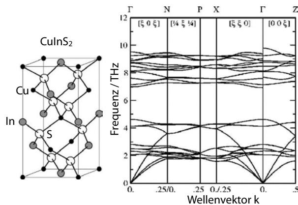
Abbildung 4.33: Phononenspektrum für CuInS 2 .
