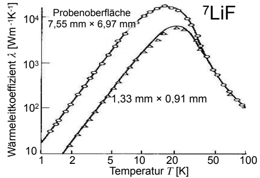
Abbildung 4.81: Temperaturabhängigkeit des Wärmeleitkoeffizienten in unterschiedlichen Proben.
