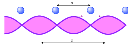
Abbildung 4.9: Reflexion einer Welle, welche die Bragg-Bedingung \lambda = 2a erfüllt.
