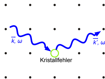
Abbildung 4.75: Streuung eines Phonons an einem Gitterfehler.
