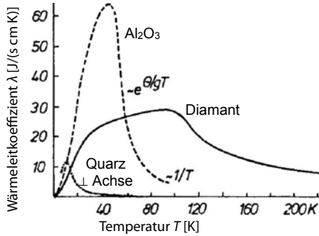
Abbildung 4.80: Temperaturabhängigkeit des Wärmeleitkoeffizienten.
