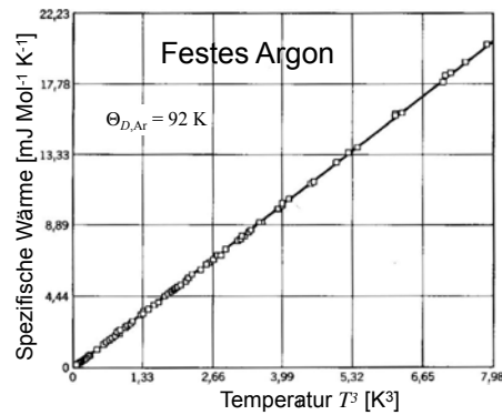
Abbildung 4.56: Wärmekapazität von festem Argon bei tiefer Temperatur.
