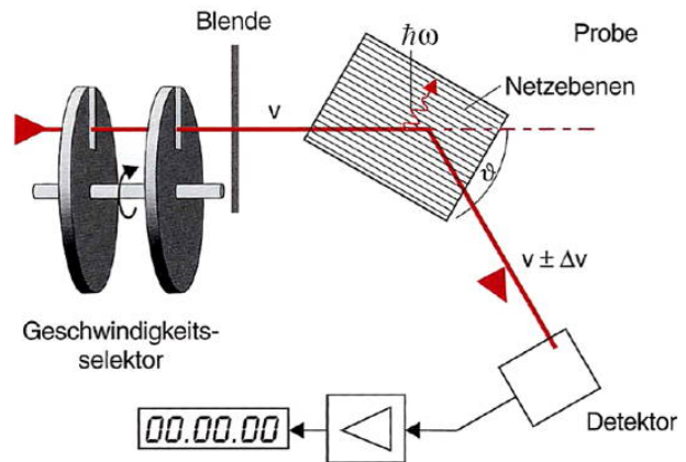
Abbildung 4.42: Flugzeit-Spektrometer für Neutronen.
