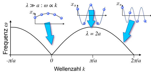
Abbildung 4.3: Dispersion der eindimensionalen Kette.
