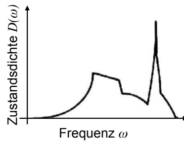
Abbildung 4.60: Reale Zustandsdichte.
