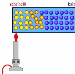
Abbildung 4.71: Wärmeleitung.
