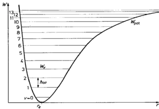
Abbildung 4.67: Anharmonisches Potenzial.
