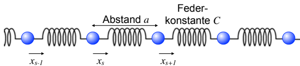
Abbildung 4.2: Eindimensionale Kette.
