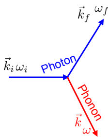
Abbildung 4.36: Inelastische Lichtstreuung.
