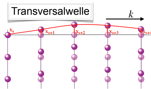
Abbildung 4.24: Transversalwelle.
