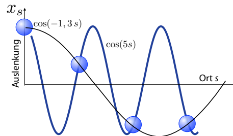
Abbildung 4.4: Zwei Schwingungen mit unterschiedlichen Wellenzahlen, welche die gleiche Auslenkung der Atome ergeben.
