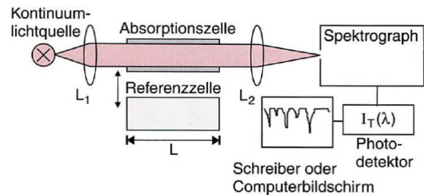
Abbildung 4.34: Prinzip der Infrarotspektroskopie.
