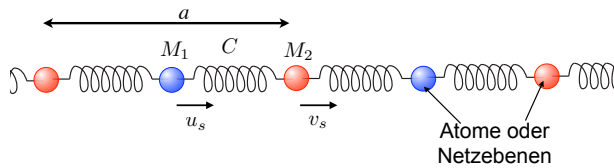
Abbildung 4.26: Eindimensionale Kette mit 2 Atomen pro Elementarzelle.
