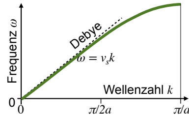
Abbildung 4.52: Vereinfachte Dispersion im Debye-Modell.
