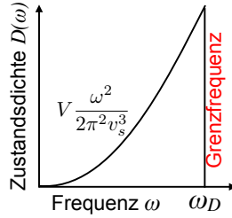
Abbildung 4.53: Zustandsdichte im Debye-Modell.
