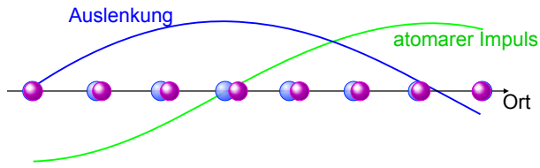
Abbildung 4.46: Auslenkung und Impuls der Gitteratome.
