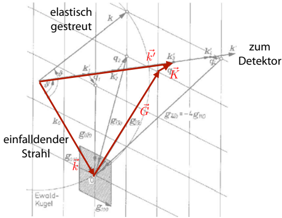
Abbildung 4.40: Impulse beim inelastischen Streuprozess.
