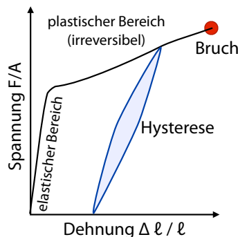
Abbildung 4.15: Elastische vs. plastische Verformung.
