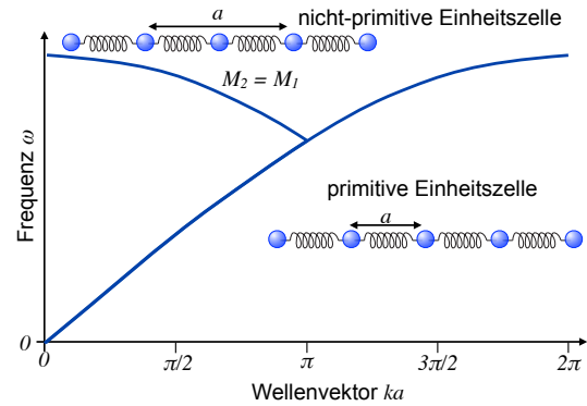
Abbildung 4.30: Faltung der Dispersionsrelation bei Verdoppelung der Einheitszelle.
