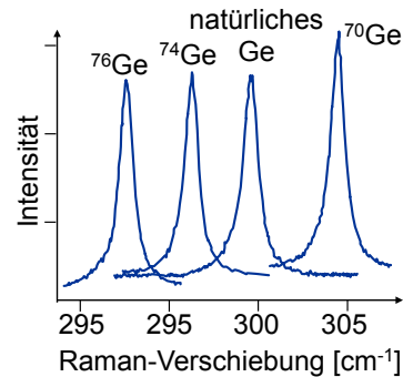
Abbildung 4.39: Raman-Streuung an Germanium mit unterschiedlichen Atommassen.
