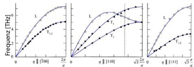
Abbildung 4.31: Phononenspektrum für Kupfer.
