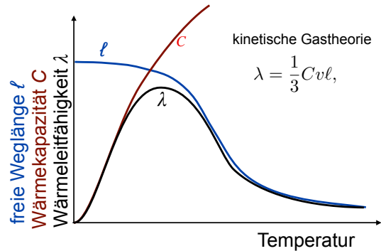
Abbildung 4.79: Beiträge zur Wärmeleitung.
