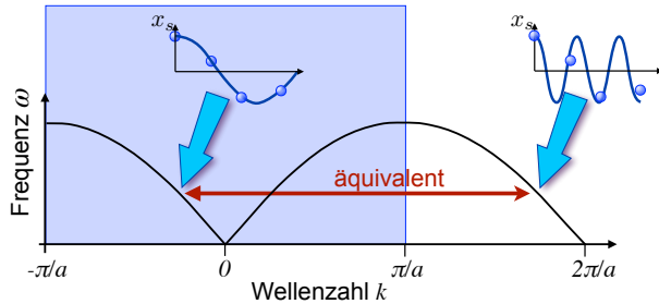
Abbildung 4.5: Die 1. Brillouin-Zone enthält die gesamte Information.
