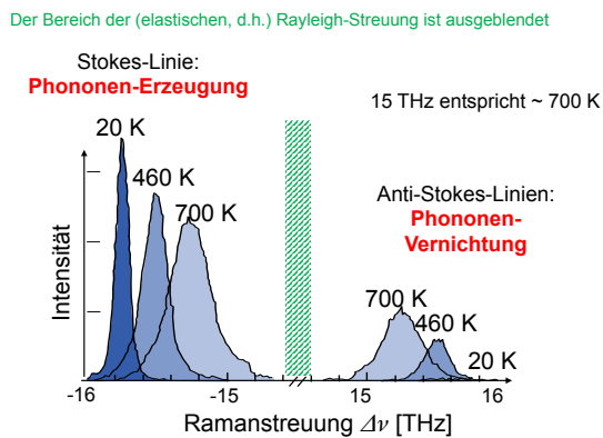
Abbildung 4.38: Raman-Streuung an Silizium.
