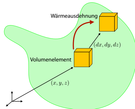
Abbildung 4.69: Wärmeausdehnung.
