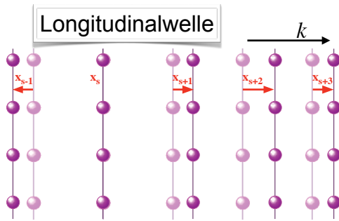
Abbildung 4.23: Longitudinalwelle.
