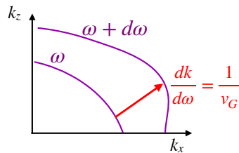
Abbildung 4.62: Iso-Frequenzflächen und Gruppengeschwindigkeit.
