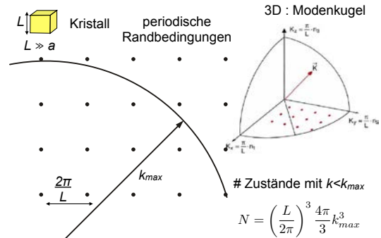
Abbildung 4.51: Zustände im k -Raum.
