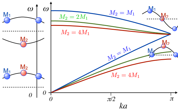
Abbildung 4.29: Einfluss des Massenverhältnisses M_2/M_1 auf den akustischen und optischen Ast.
