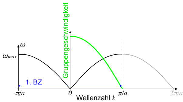
Abbildung 4.8: Dispersion von Frequenz und Gruppengeschwindigkeit.
