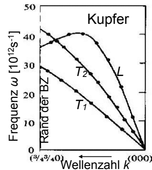
Abbildung 4.25: Dispersion von Kupfer: longitudinale und transversale Zweige.
