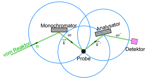
Abbildung 4.41: 3-Achsens Neutronenspektrometer.
