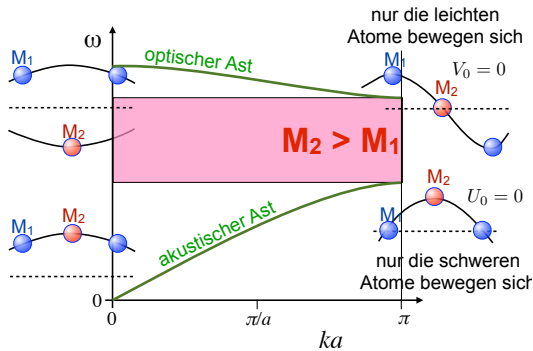
Abbildung 4.27: Auslenkung der Atome im akustischen und optischen Ast.
