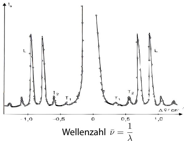
Abbildung 4.37: Brillouin-Spektrum von SbSi.
