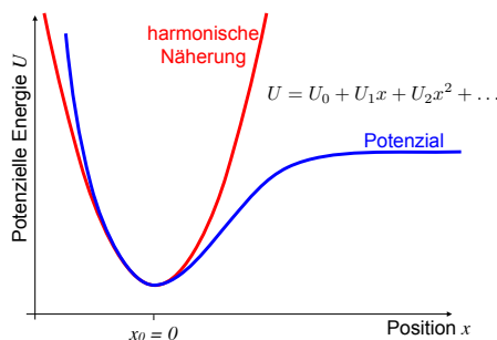
Abbildung 4.1: Potenzialverlauf und harmonische Näherung.
