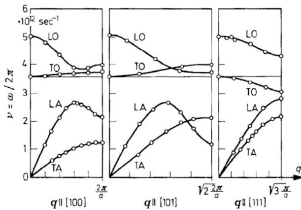
Abbildung 4.32: Dispersion der Schwingungsmoden in KBr.
