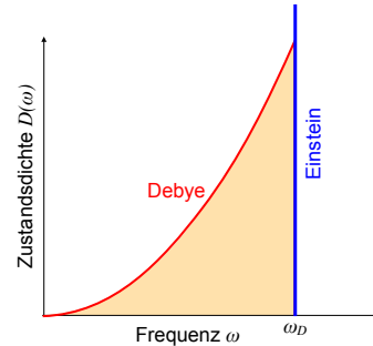
Abbildung 4.57: Vergleich der Zustandsdichten in den Modellen von Einstein und Debye.
