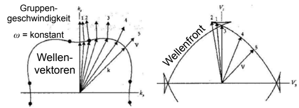
Abbildung 4.19: Links: Oberfläche konstanter Frequenz im k -Raum und zugehörige Gruppengeschwindigkeitsvektoren. Rechts: Wellenfront und Ausbreitungsrichtung.
