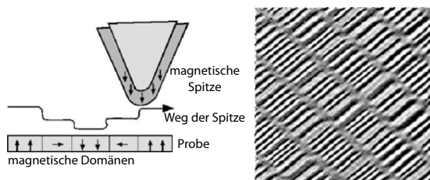
Abbildung 8.90: Links: Prinzip der magnetischen Kraftmikroskopie. Rechts: Strukturen auf einer Festplatte.
