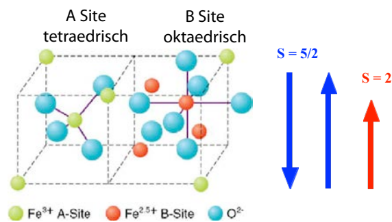
Abbildung 8.64: Struktur und magnetische Ordnung in \text{Fe}_2\text{O}_3 .
