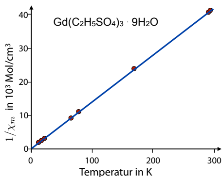
Abbildung 8.18: Kehrwert der magnetischen Suszeptibilität als Funktion der Temperatur.
