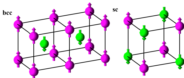
Abbildung 8.60: Antiferromagnetische Ordnung im bcc und sc Gitter.
