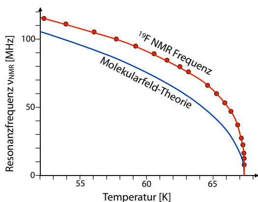
Abbildung 8.70: Resonanzfrequenz der 19 F Kernspins in MnF 2 als Funktion der Temperatur.
