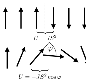
Abbildung 8.78: Wechselwirkungsenergie im Bereich der Domänenwand.
