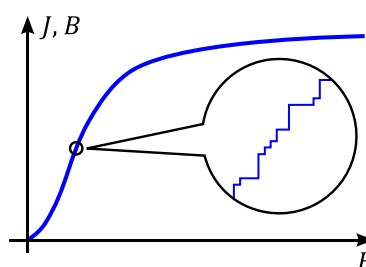
Abbildung 8.86: Sprunghafte Änderung der Magnetisierung.
