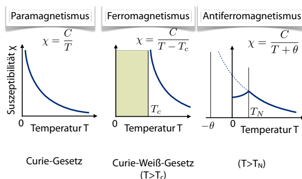
Abbildung 8.66: Temperaturabhängigkeit der Suszeptibilität für unterschiedliche magnetische Ordnung.
