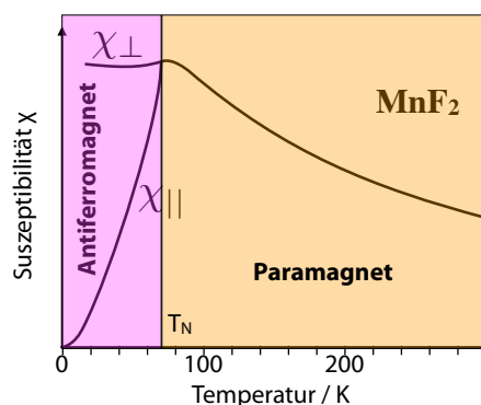
Abbildung 8.68: Anisotrope Suszeptibilität als Funktion der Temperatur.
