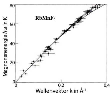
Abbildung 8.69: Magnonendispersion in RbMnF 3 .
