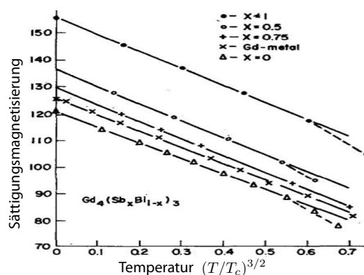
Abbildung 8.58: Spontanmagnetisierung als Funktion der Temperatur und Bloch'sches T^{3/2} -Gesetz.
