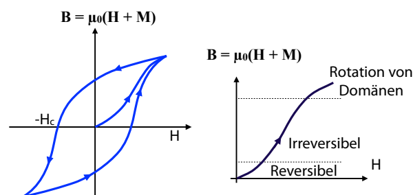
Abbildung 8.87: Links: magnetische Hysterese. Rechts: Reversibles vs. irreversibles Verhalten.
