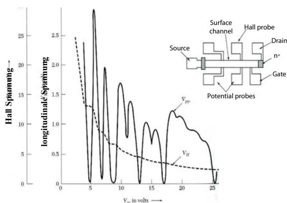
Abbildung 8.38: Messprinzip und Messresultate für den ganzzahligen Quanten-Hall Effekt.
