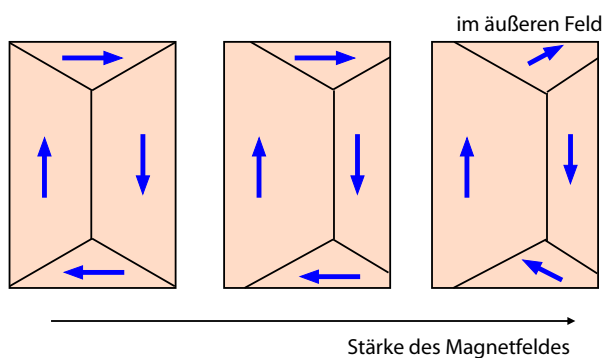
Abbildung 8.85: Wandern von Domänen im Magnetfeld.
