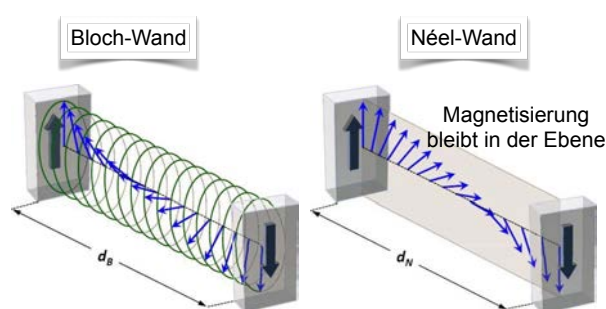
Abbildung 8.83: Bloch-Wand vs. Néel-Wand.
