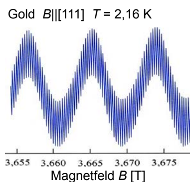
Abbildung 8.36: deHaas-van Alphen Oszillationen von Gold in \langle 111 \rangle -Richtung und die zugehörigen Bahnen auf der Fermifläche.
