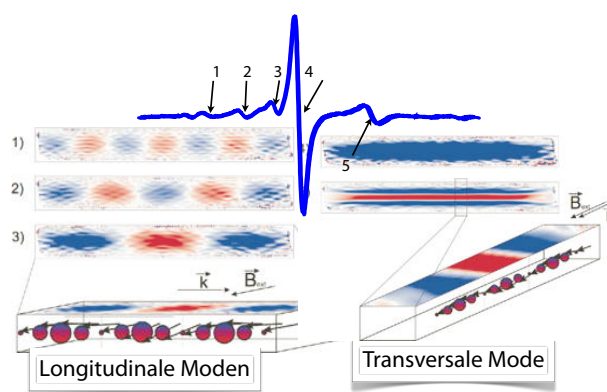
Abbildung 8.56: Gemessenes FMR Spektrum und Simulierte Spin-Wellen.
