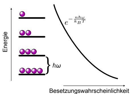
Abbildung 8.57: Thermische Besetzung von Magnonzuständen.
