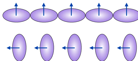
Abbildung 8.80: Ursprung der Anisotropie der Austausch-Wechselwirkung.
