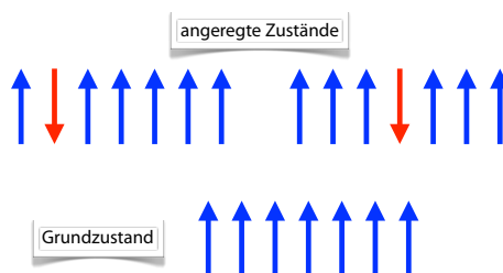
Abbildung 8.47: Angeregte Spinzustände.
