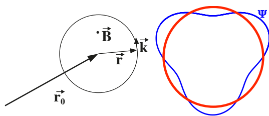
Abbildung 8.26: Links: Kreisbahn senkrecht zum Magnetfeld. Rechts: Bahn-Quantisierung.
