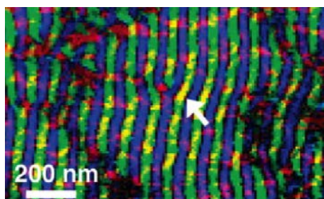
Abbildung 8.73: Helikale Spinordnung in \text{Fe}_{0.5}\text{Cr}_{0.5}\text{Si} .
