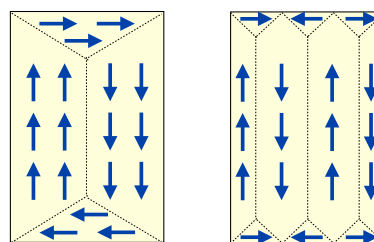
Abbildung 8.77: Oberflächennahe Domänen.
