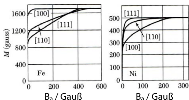
Abbildung 8.82: Asymmetrische Magnetisierungskurven in Fe und Ni.
