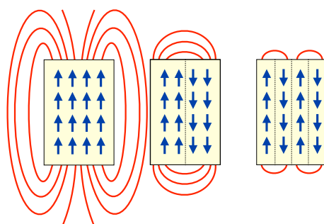
Abbildung 8.76: Reduktion der magnetischen Feldenergie durch Domänenbildung.
