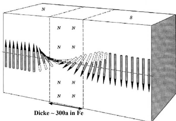
Abbildung 8.79: Änderung der Spin-Orientierung im Bereich der Bloch-Wand.
