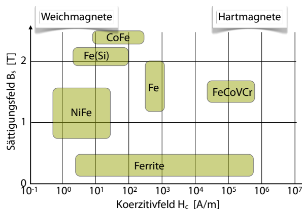
Abbildung 8.89: Übersicht über die magnetischen Eigenschaften unterschiedlicher Werkstoffe.
