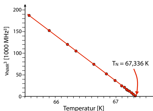
Abbildung 8.71: Resonanzfrequenz der 19 F Kernspins in MnF 2 als Funktion der Temperatur.
