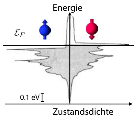
Abbildung 8.22: Zustandsdichte und Ferminiveau für die Subbänder von Ni. [2]
