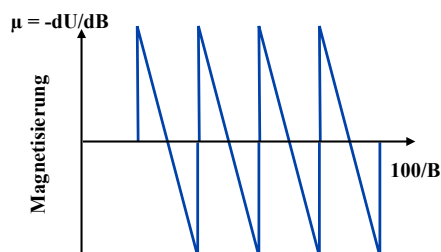
Abbildung 8.34: Oszillatorische Abhängigkeit der Magnetisierung von der inversen Magnetfeldstärke.
