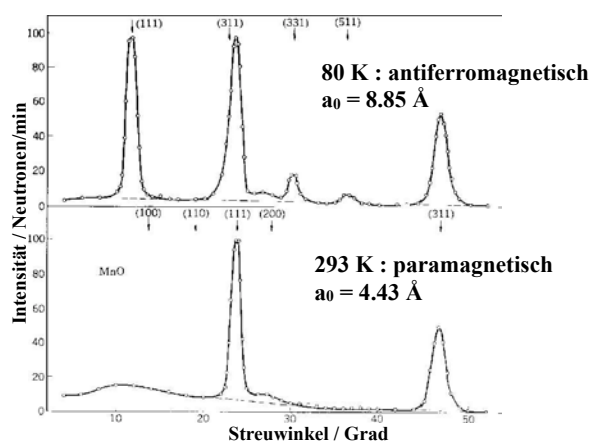
Abbildung 8.63: Magnetische Neutronen-Beugung gemessen an \text{MnO}_2 . Oben: antiferromagnetische Ordnung bei 80 K. Unten: paramagnetische Ordnung bei 293 K.
