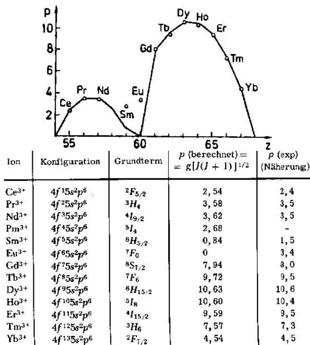
Abbildung 8.12: Effektive Magnetonzahlen für die Lanthaniden.
