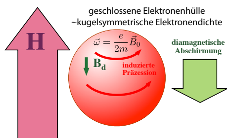
Abbildung 8.4: Diamagnetische Abschirmung.
