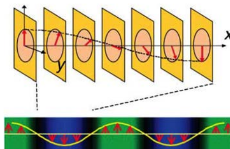
Abbildung 8.72: Helikale Spinordnung.
