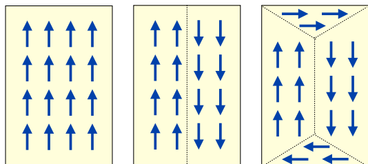
Abbildung 8.74: Magnetische Domänen.
