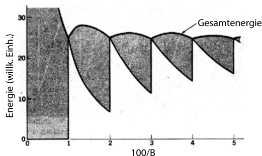
Abbildung 8.33: Gesamte Energie der besetzten Landauzustände als Funktion der Magnetfeldstärke.
