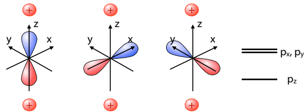
Abbildung 8.13: Aufhebung der Entartung durch asymmetrische Ladungsverteilung.
