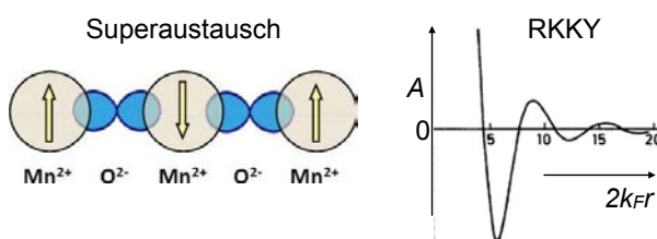
Abbildung 8.42: Indirekte Austauschwechselwirkung.
