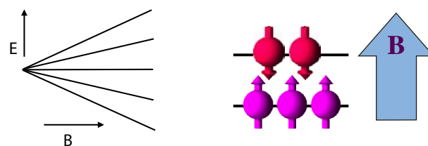
Abbildung 8.16: Energie und Besetzungszahlen der Spin-Zustände im Magnetfeld.
