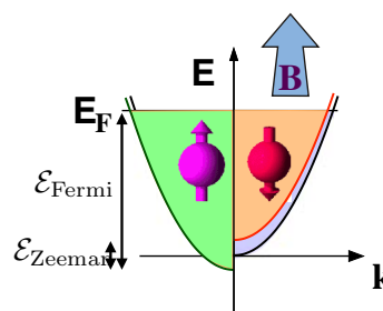
Abbildung 8.21: Verschiebung der Spinzustände von freien Elektronen im Magnetfeld.
