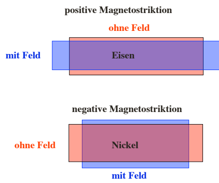
Abbildung 8.93: Magnetostruktion.
