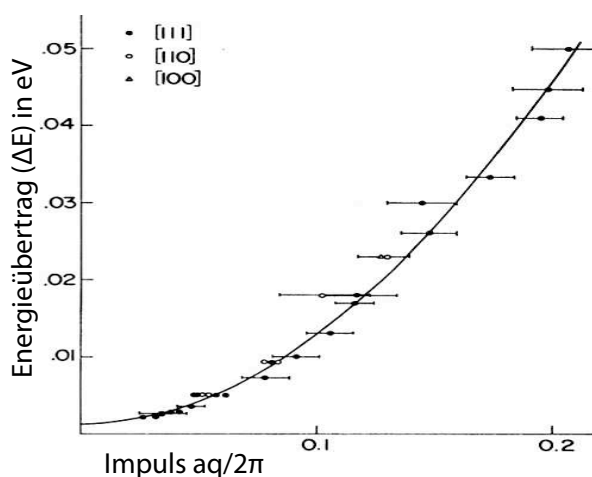
Abbildung 8.53: Dispersionsrelation der Spinwellen in \text{Co}_{92}\text{Fe}_8 . [8]
