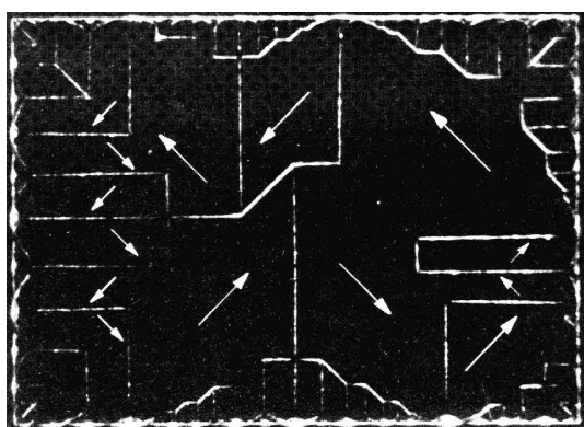
Abbildung 8.81: Ferromagnetische Domänen in einem Ni-Plättchen.
