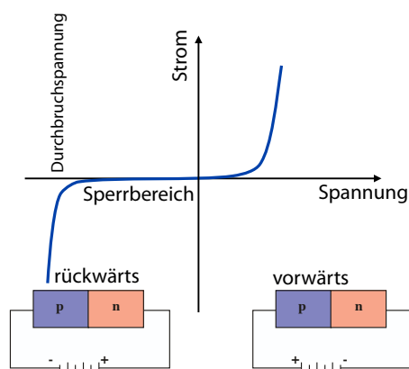
Abbildung 7.54: Strom-Spannungskennlinie einer typischen Diode.
