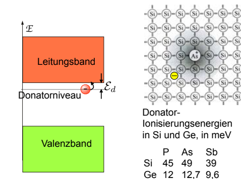
Abbildung 7.39: Energie und Struktur eines Donator-Zentrums.
