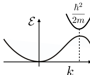
Abbildung 7.18: Bandkrümmung am Zonenrand.
