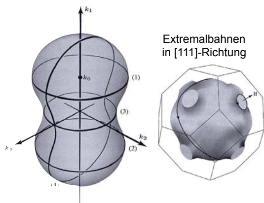
Abbildung 7.29: Extremalbahnen für unterschiedliche Magnetfeldrichtungen.
