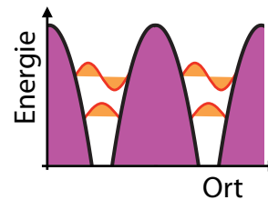
Abbildung 7.26: Lokalisierung von elektronischen Zuständen in Potenzialminima.
