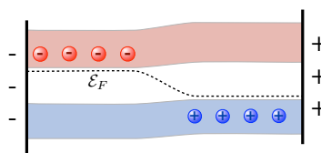
Abbildung 7.53: Sperrschicht bei Anlegen einer Spannung in Vorwärtsrichtung.
