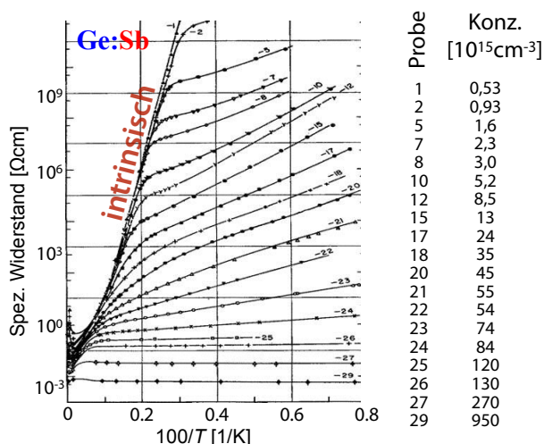
Abbildung 7.37: Einfluss von Dotierung und Temperatur auf den spezifischen Widerstand. [2]
