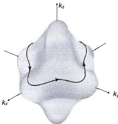
Abbildung 7.27: Bahn eines Elektrons im k -Raum.
