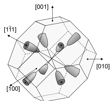
Abbildung 7.20: Ellipsoide konstanter Energie für Germanium am L-Punkt, d.h. in [111]-Richtung.
