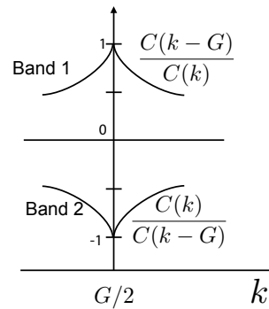
Abbildung 7.22: Koeffizienten der Zustände am Zonenrand.
