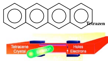
Abbildung 7.5: Tetracene als organischer Halbleiter.
